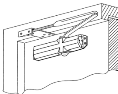
ukázka montáže s paralelním ramenem
