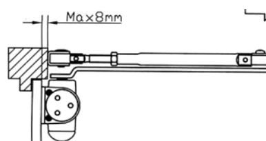
montáž s běžným ramenem
