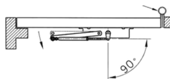
montáž s paralelním ramenem
