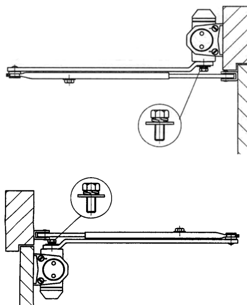
ukázky montáže na rám dveří a na dveřní křídlo
