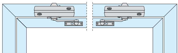
Montáž na dveře
